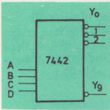
Fig. 45. Decodificator binar-zecimal
