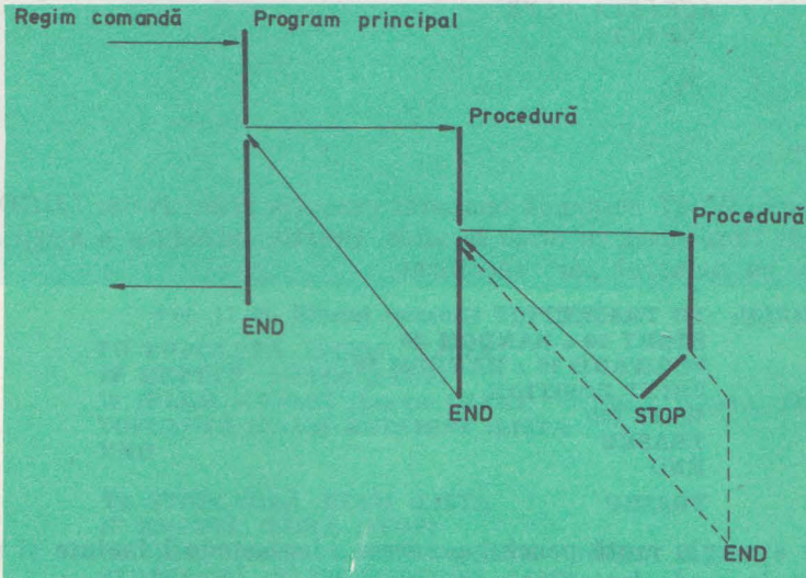
Fig. 11.27. Efectul comenzii STOP
