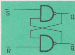
Fig. 4.8. Bistabil realizat cu circuite SI-NU (NAND) și tabela de adevăr
