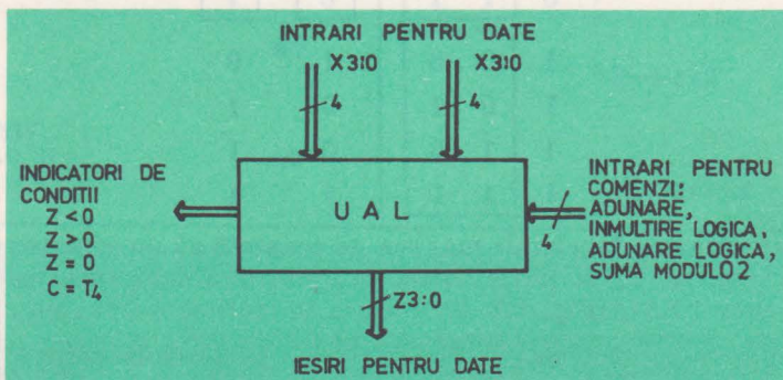
Fig. 4.4. Unitate aritmetică-logică pentru numere binare de 4 biți
