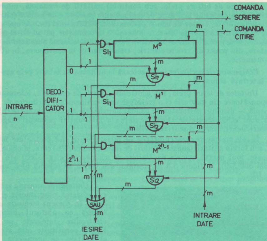
Fig. 5.4. Modelul funcțional al unei memorii interne
