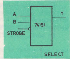
Fig. 4.6. Multiplexor 2 : 1
