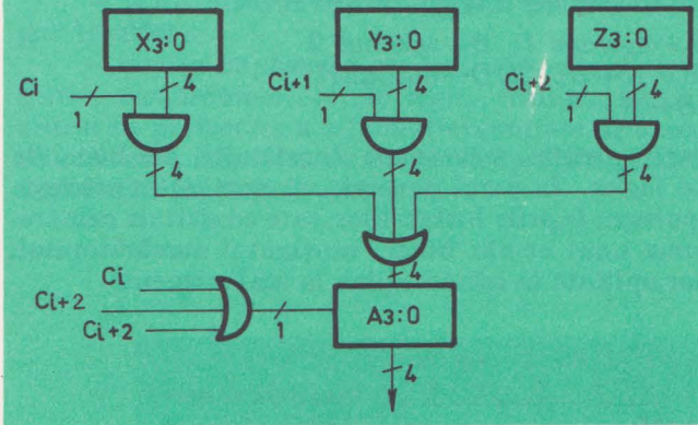
Fig. 4.11. Încărcarea unui registru de la mai multe surse de informații
